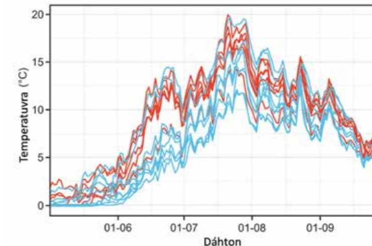
Govus b. Čáhce temperatuvrra profilat vihttanuppelohkái jogain gos leat mihtidan temperatuvrraid 2020 geassemánu rájes golggotmánu šaddoáigodaga rádjai. Rukses ja alit linjjat mearkašit jogaid gos gávnnaimet T. bryosalmonae ( Rukses ) ja ( alit ) gos eai gávdnan njoammuma
