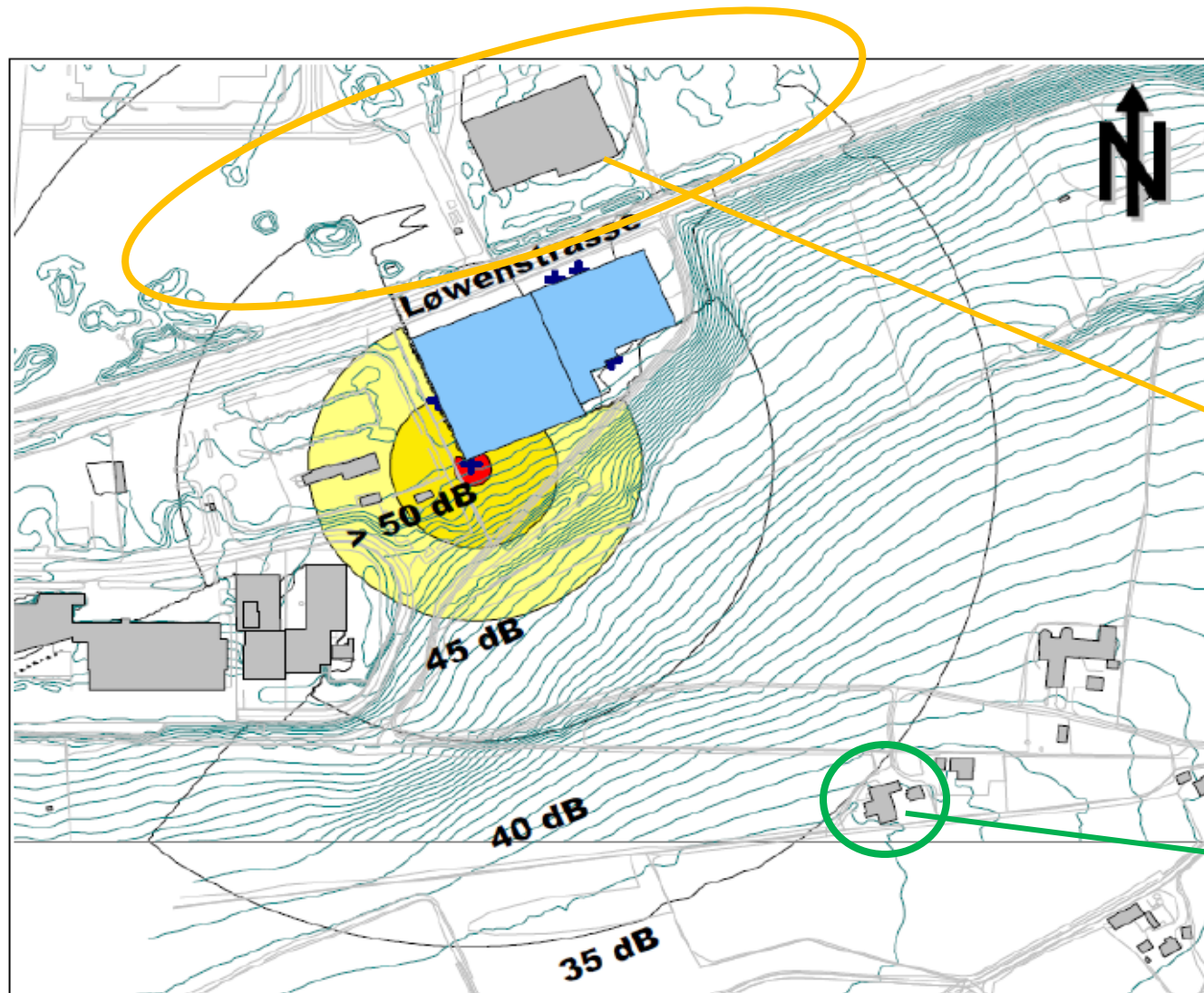
Figur 4-2: Støyberegning L_{Night} 4 meter over terrenget med lydeffektnivå L_{WA} = 97 dB for skorsteinsutløp med alle andre støykilder i tabell 3-4 i drift i nattperioden. Figuren angir støykoter med gul og rød sone iht. krav i T-1442 for støy fra industri. Til informasjon er vist utvidede støykoter for støy fra tekniske installasjoner i NS 8175 klasse C for 40 og 35 dB som sorte sirkler. I NS 8175 er nattkravet til støy 35 dB. Eksempel på relevant nattkrav i NS 8175 er støy fra ventilasjonsanlegg i en boligblokk over på en annen. Blå kryss markerer plassering av støykilder: Se også figur 3-2.
