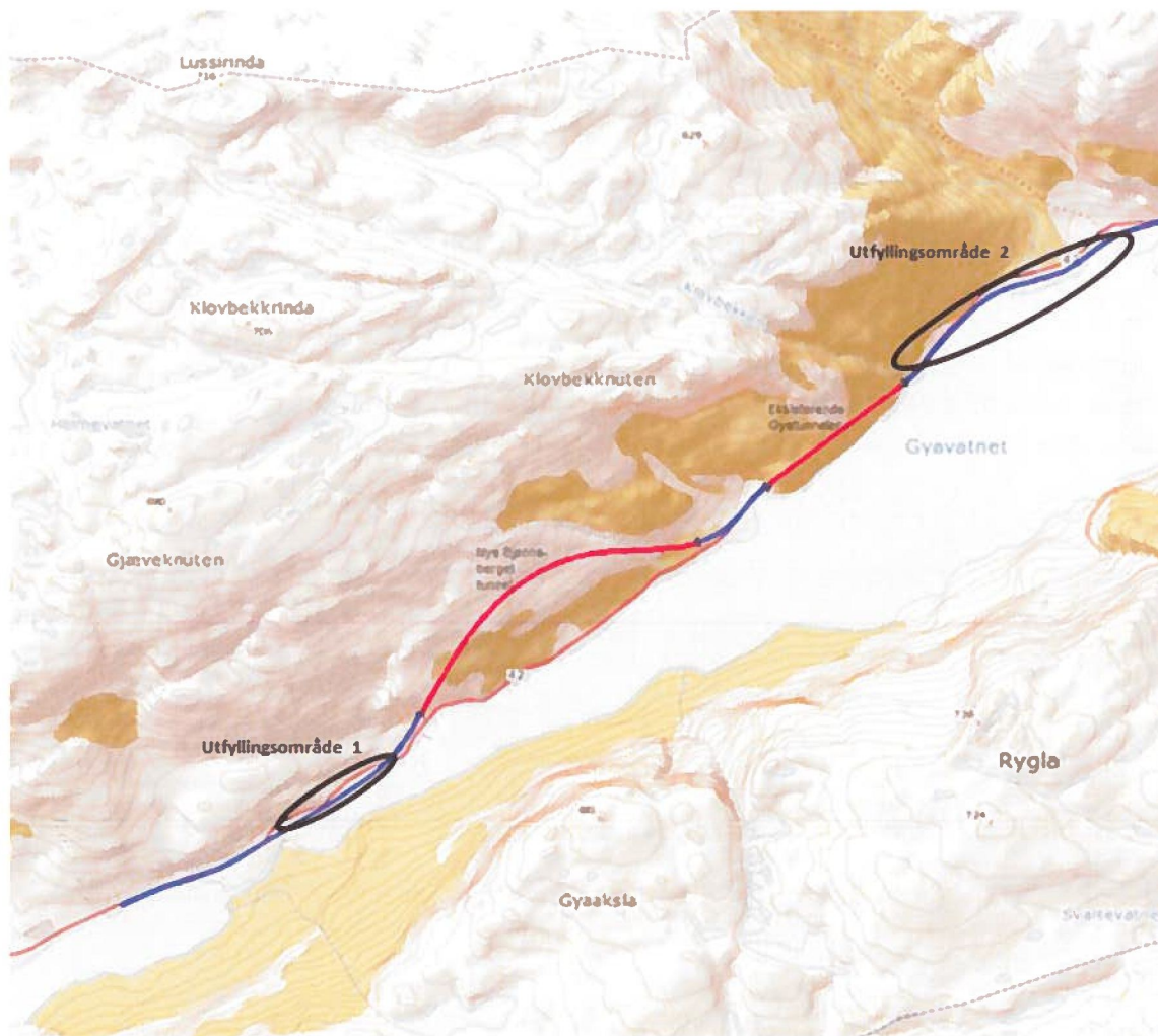
Figur 2. Oversiktskart. Ny veg er vist med blått. Eksisterende vei og ny tunnel er vist med rødt. Svart markerer planlagte utfyllingsområder.
