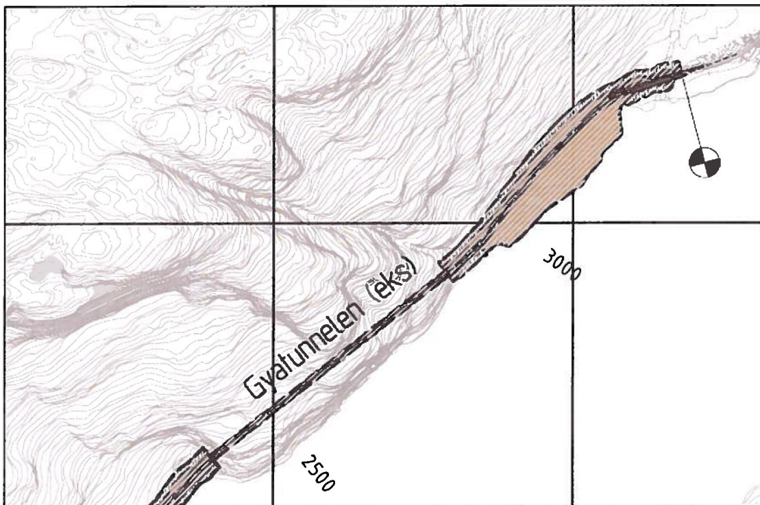
Figur 4. Utsnitt fra godkjent reguleringsplan som viser fylling i østre del av Gyavatnet.
