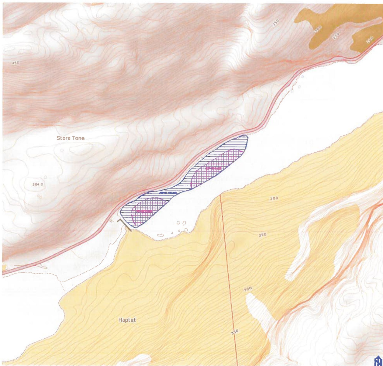
Figur 6. Kart over område som er planlagt mudret. Lilla skravur er minimumsareal som skal mudres. Blå skravur viser grense for maksimumsareal som skal mudres.
