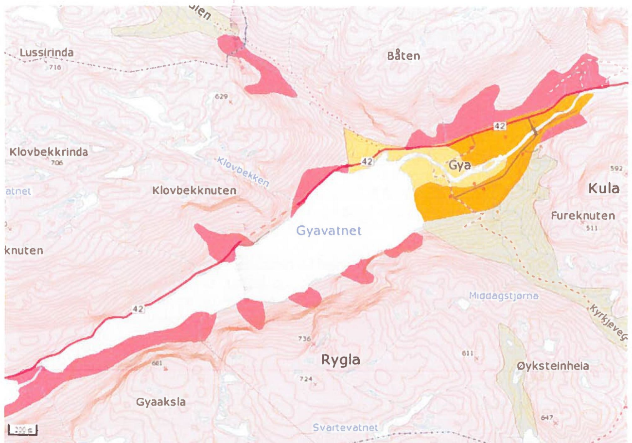
Figur 6: Løsmasser rundt Gyavatnet (NGU). Røde felter er skredmateriale, rosa bart fjell/grunnlendt. Orange er brelvavsetninger og gult er elveavsetninger
