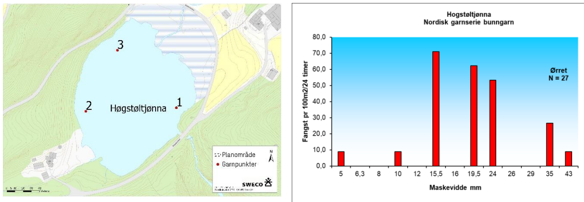
Figur 0-16. Resultat fra prøvefiske i Høgstøltjønna høsten 2020 med nordiske oversiktsgarn. Figuren viser antall fisk fanget pr. maskeviddestørrelse.
