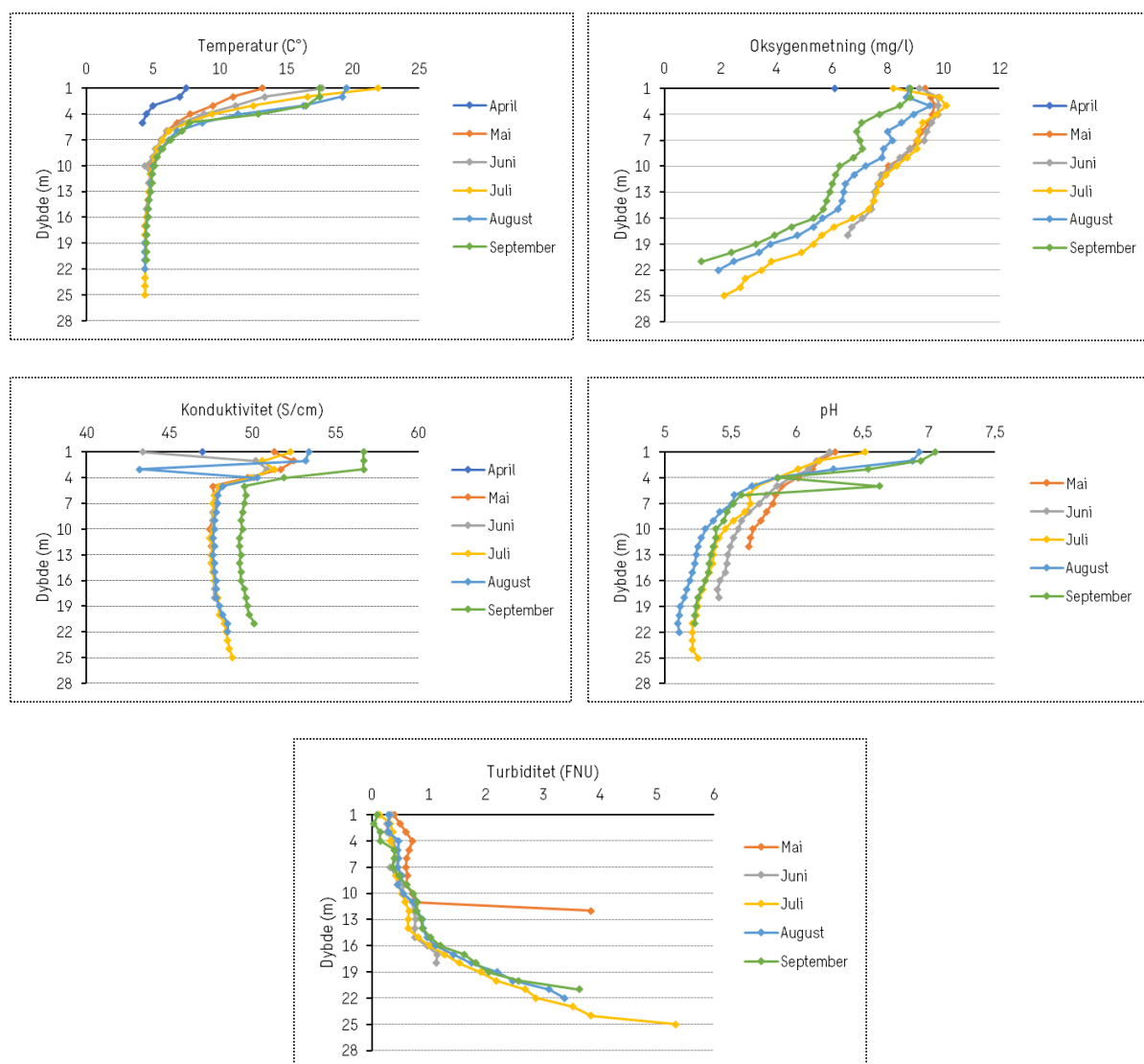
Figur 0-15. Temperatur, oksygen, konduktivitet, pH og turbiditet målt månedlig sommeren 2021 pr. dybdemeter i Unndalstjønna.
