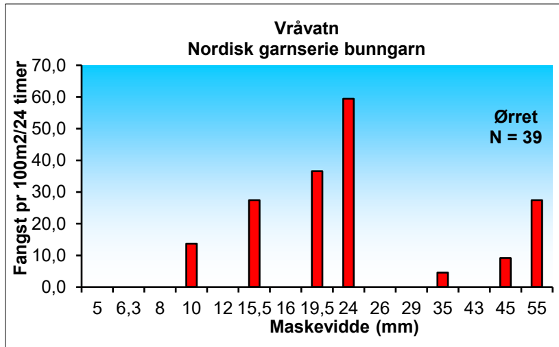
Figur 0-21. Resultater fra prøvofiske gjennomført i Vråvatn høsten 2020.
