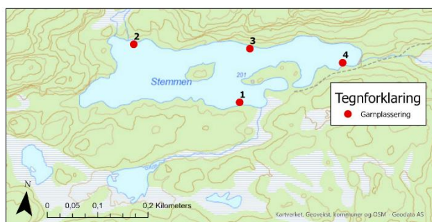
Figur 0-20. Høyre: plassering av garn i Stemmen under prøvefisket høsten 2020. Venstre bilde: ørret fanget i Stemmen. Gyteklar hannørret. Foto: Sweco.
