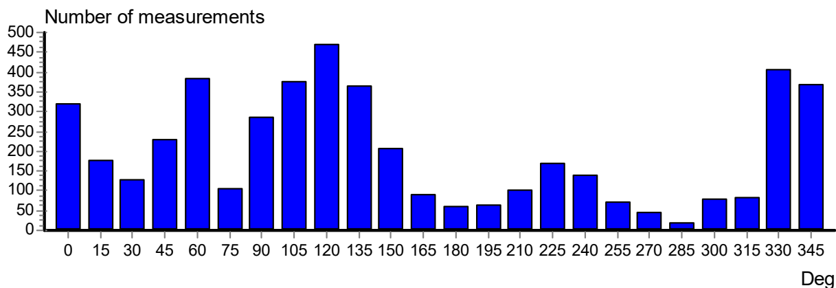
Figur 4: Antall registreringer pr 15° sektor. Registreringene er foretatt ved 12 m dyp ved resipienten for utslippsområdet fra Lødingen Fisk AS, Bresja, i Lødingen kommune, Nordland.
