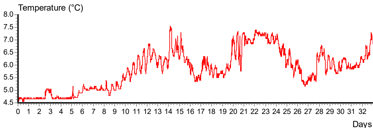
Figur 1: Temperaturutvikling i registreringsperioden ved 12 m dyp ved resipienten for utslippsområdet fra Lødingen Fisk AS, Bresja, i Lødingen kommune, Nordland.
