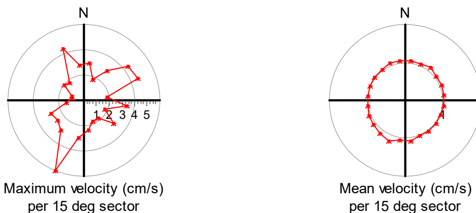
Figur 6: Fordelingsdiagram som viser fordeling av strømaktivitet i de forskjellige sektorer (pr 15°). Diagrammet til venstre viser maksimal strømshastighet registrert i perioden i den enkelte sektor. Diagrammet til høyre viser middel strømshastighet registrert i den respektive sektor for samme periode. Registreringene er foretatt ved 12 m dyp ved resipienten for utslippsområdet fra Lødingen Fisk AS, Bresja, i Lødingen kommune, Nordland.
