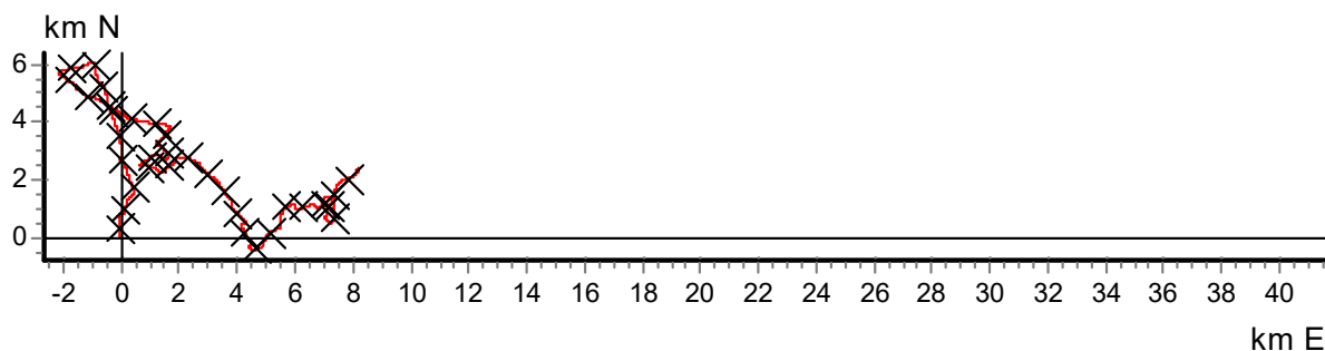
Figur 5: Vektordiagram som viser en tenkt partikkels vandring i vannmassene med utgangspunkt t=0 (ved origo) ved 12 m dyp ved resipienten for utslippsområdet fra Lødingen Fisk AS, Bresja, i Lødingen kommune, Nordland. Diagrammet viser noe turbulens og tilbakevandring i perioden.
