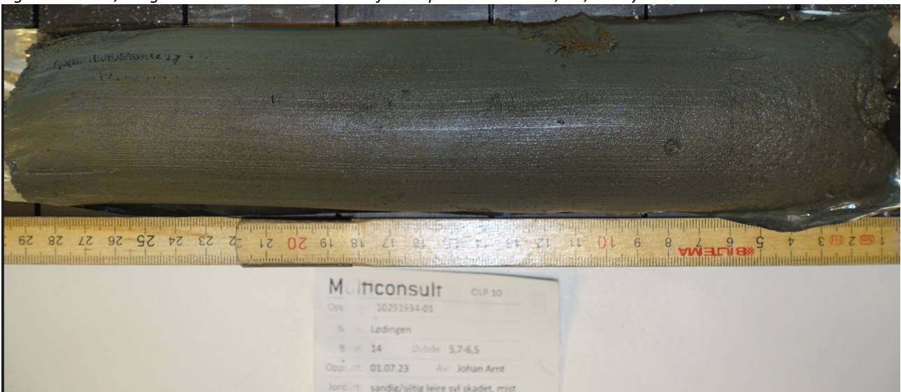
Figur 4-5: Leire, siltig fra borpunkt SW14 ved 5,7-6,5 m dybde, skadet sylinder. Denne leiren er klassifisert som leire med sprøbruddegenskaper.
