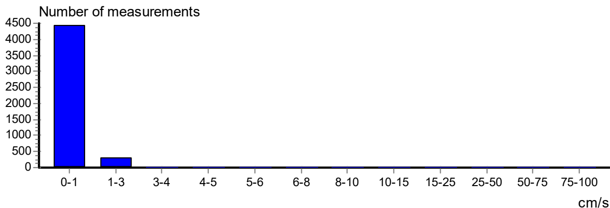
Figur 3: Antall registreringer pr strømintervall i registreringsperioden. Registreringene er foretatt ved 12 m dyp ved resipienten for utslippsområdet fra Lødingen Fisk AS, Bresja, i Lødingen kommune, Nordland. Det er flest antall registreringer i området 0-3 cm/sek.
