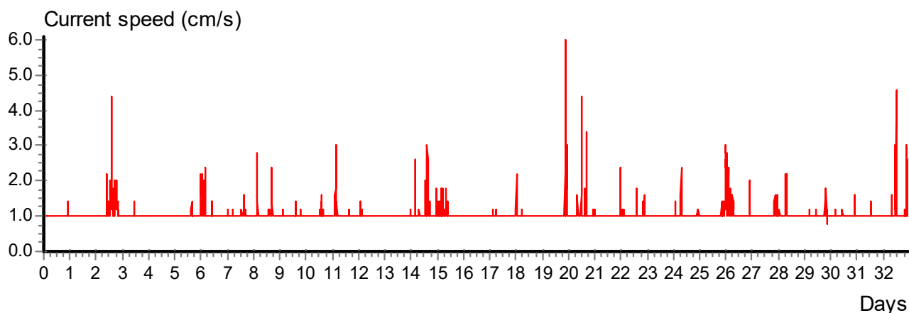
Figur 2: Strømstyrke for hver enkelt strømregistrering i perioden. Registreringene er foretatt ved 12 m dyp ved resipienten for utslippsområdet fra Lødingen Fisk AS, Bresja, i Lødingen kommune, Nordland. Vi ser at de fleste registreringer ligger i området rundt 1 cm/sek .
