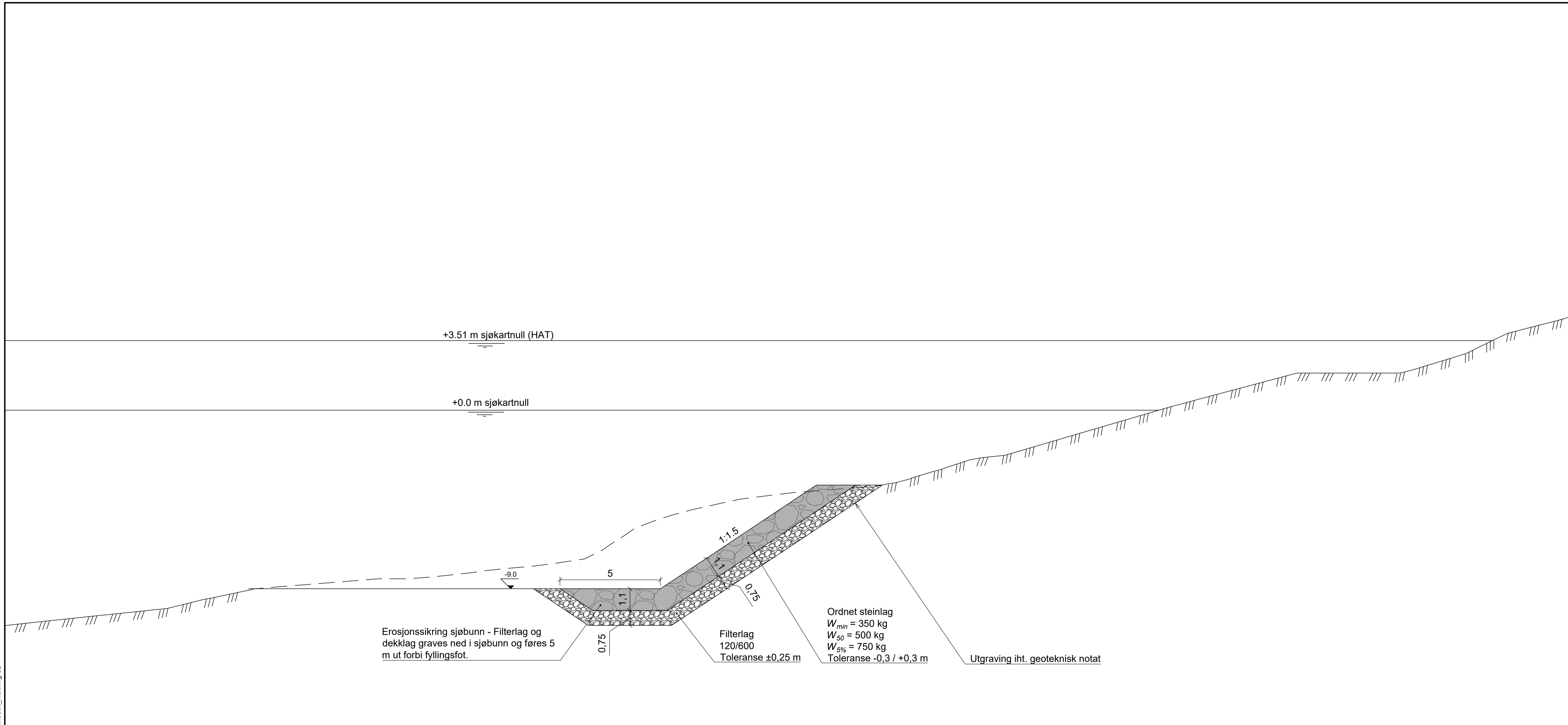
Snitt A-A
