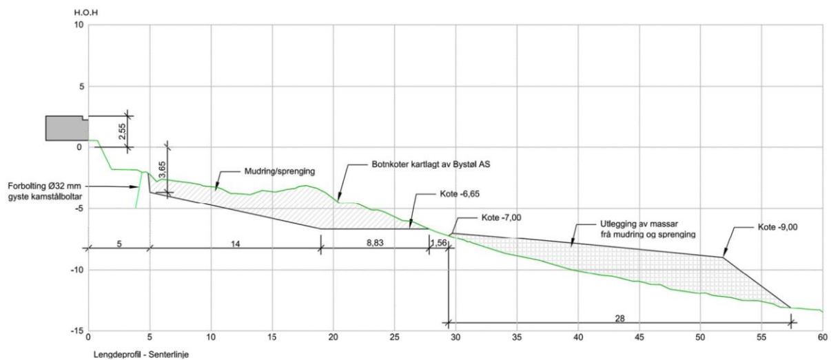
Figur 1 Lengdeprofil (Bystøl)
