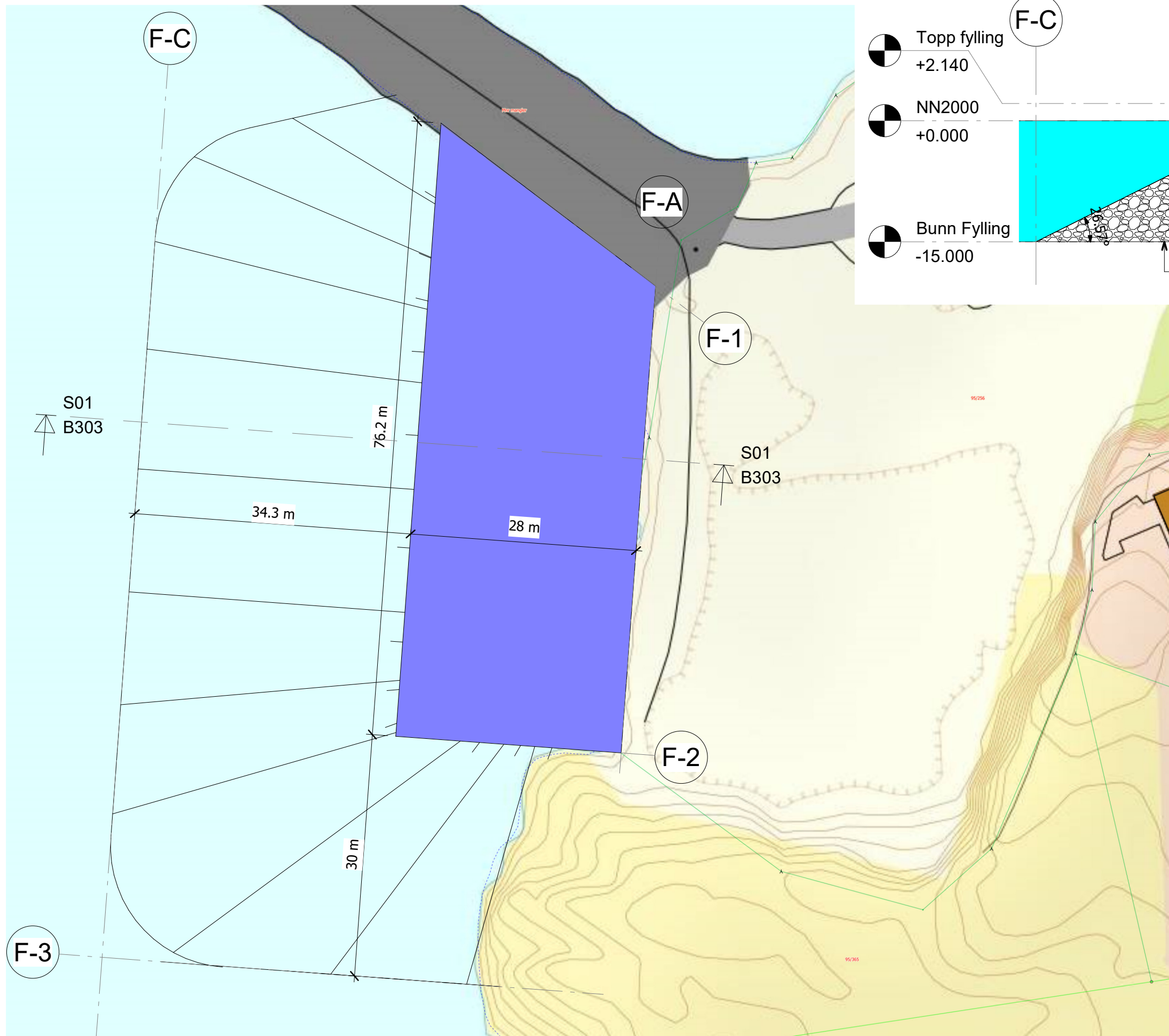
Situasjonsplan Fylling 1 : 500
