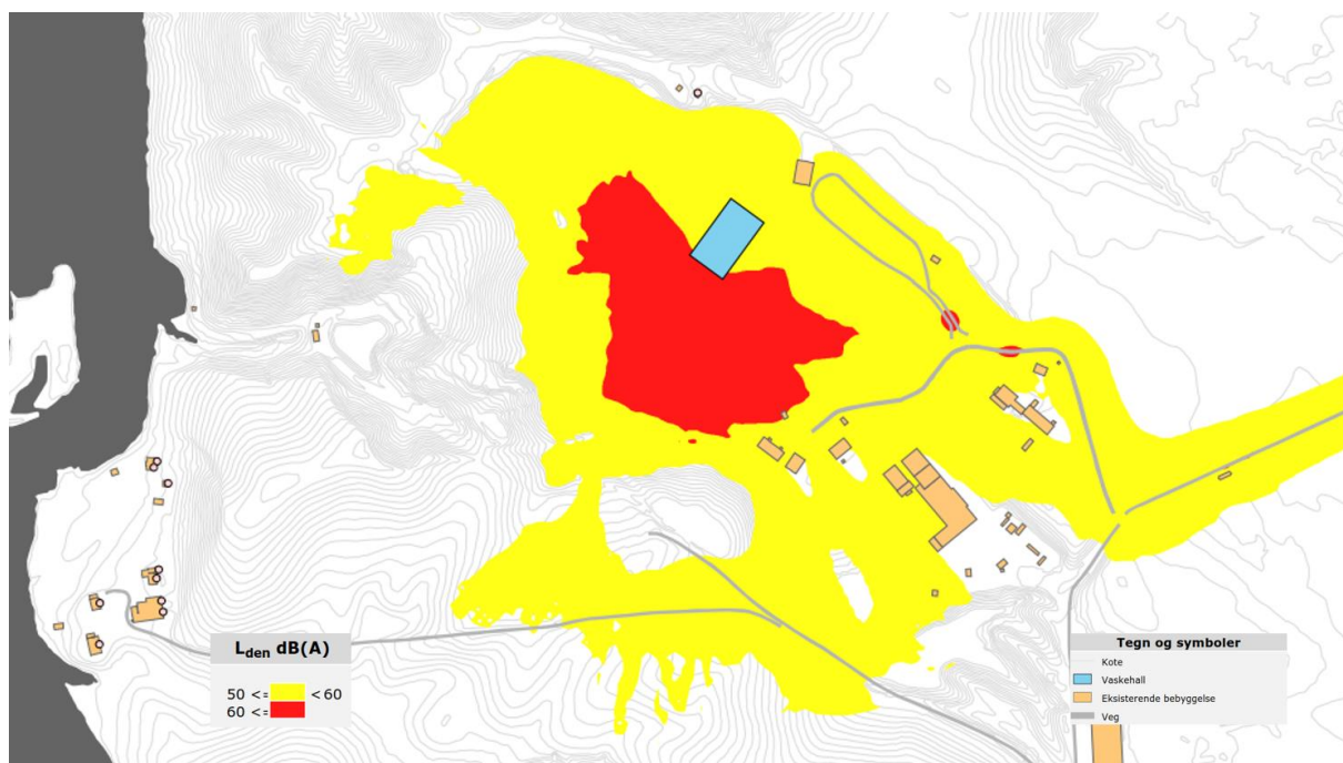
Figur 9. Støykart med beregningshøyde 4 meter.
