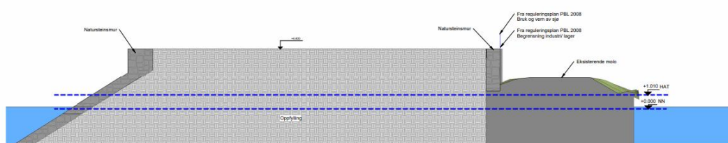
1 Snitt 1 1 : 100
